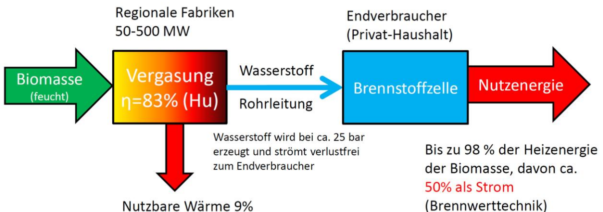
Fig. 2 Energiekette bei der thermochemischen Herstellung von Wasserstoff aus Biomasse
