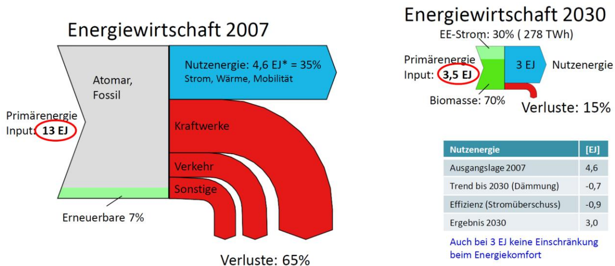
Fig. 2 Effizienz der Energiewirtschaft heute und morgen
