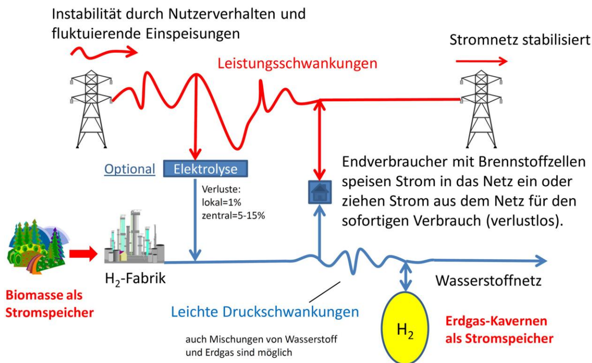
Fig. 4 Stabilisierung des Stromnetzes
